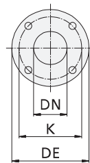
Flange Flanges
