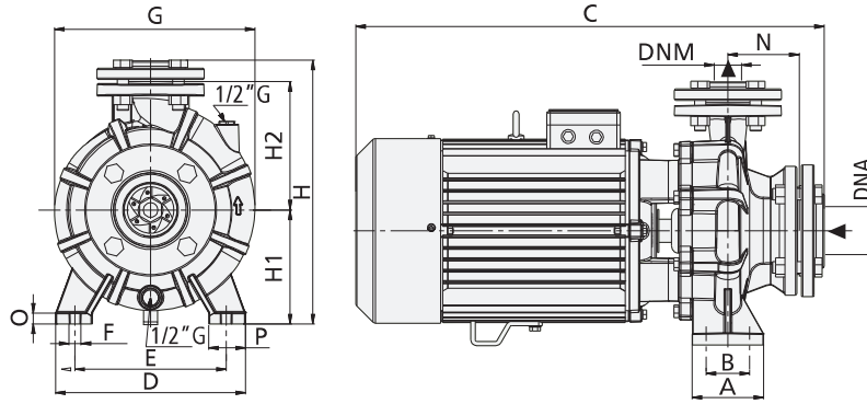
Flange Flanges
